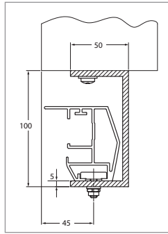
Top Fix
